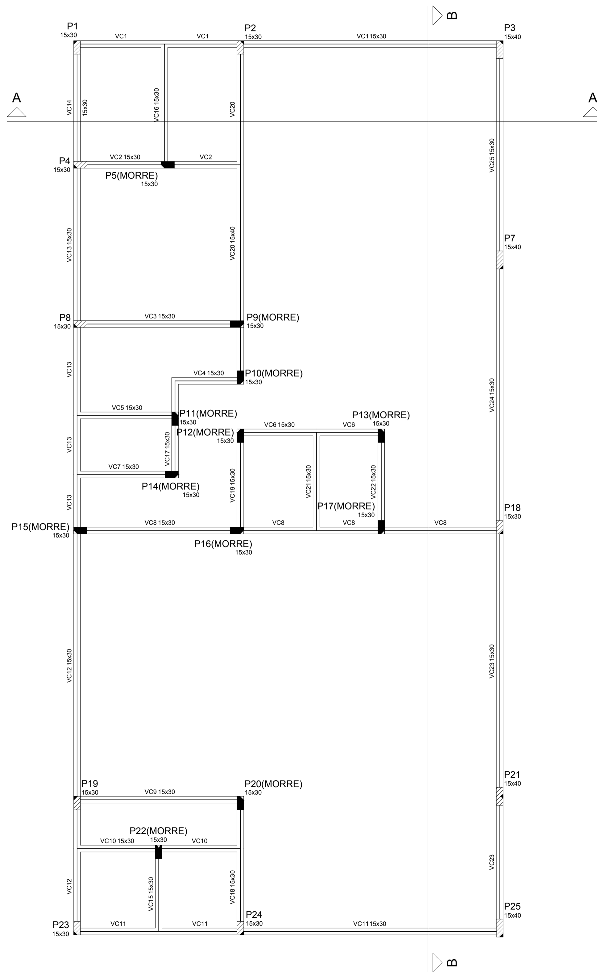
Forma do pavimento COBERTURA escala 1:50
