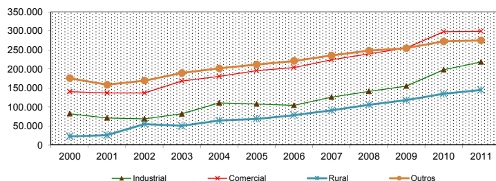
Evolução do Consumo de Energia Elétrica (MWh)
