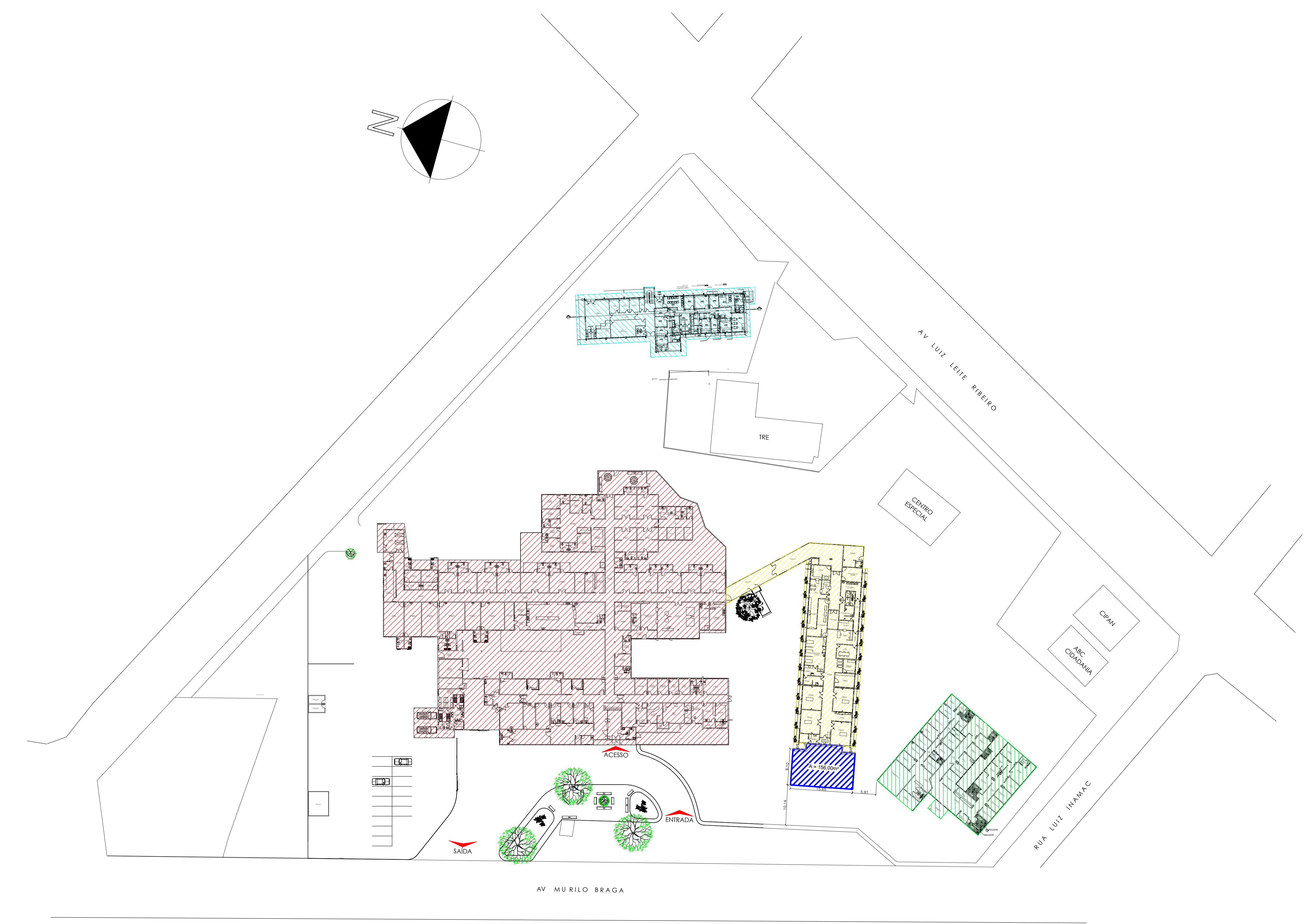
PLANTA DE LOCAÇÃO ESCALA 1/500 ■ HOSPITAL REGIONAL PORTO NACIONAL ■ HEMOCENTRO ■ CENTRO DE REABILITAÇÃO ■ CENTRO CIRÚRGICO ■ AMPLIAÇÃO
