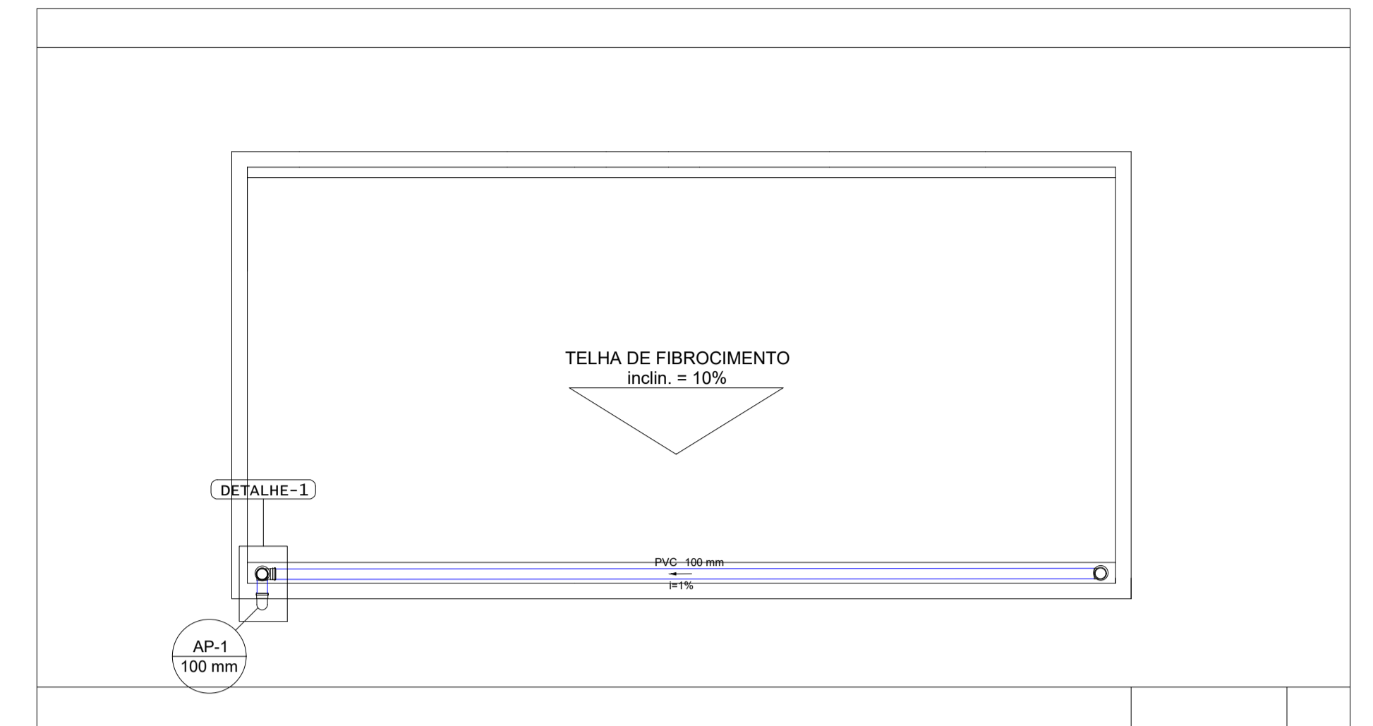
PLANTA DE COBERTURA - NECROTÉRIO ESCALA 1/50
