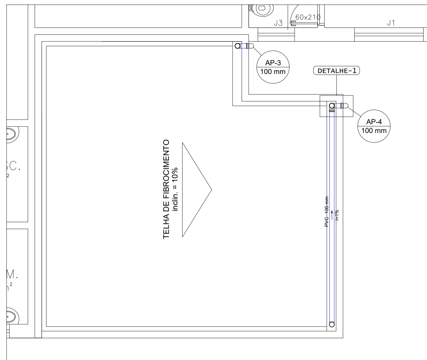
PLANTA DE COBERTURA - PRONTO SOCORRO ESCALA 1/50
