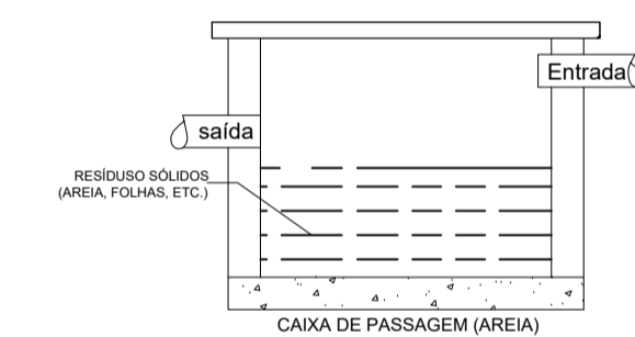
Caixa de areia pluvial SEM ESCALA
