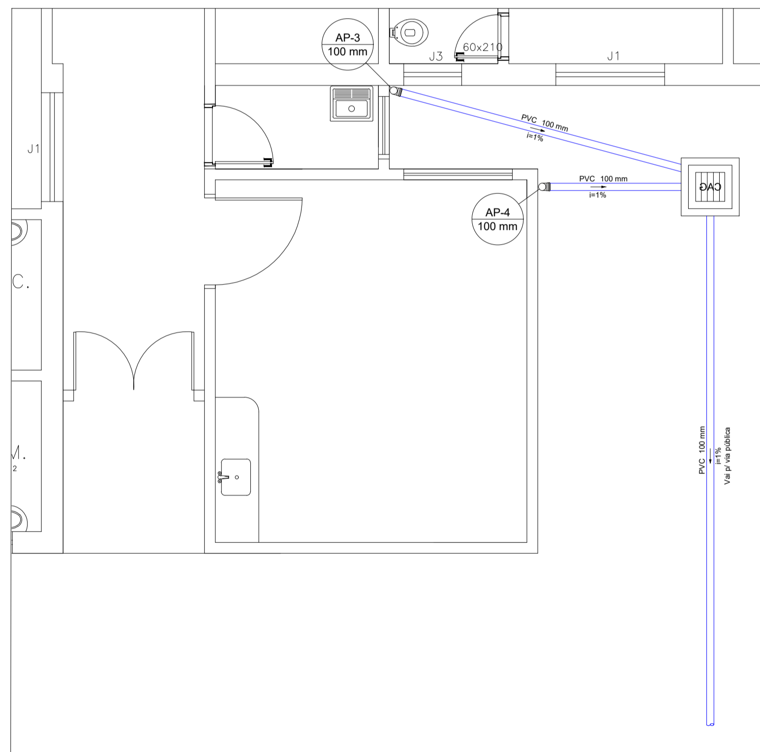
PLANTA BAIXA - PRONTO SOCORRO ESCALA 1/50
