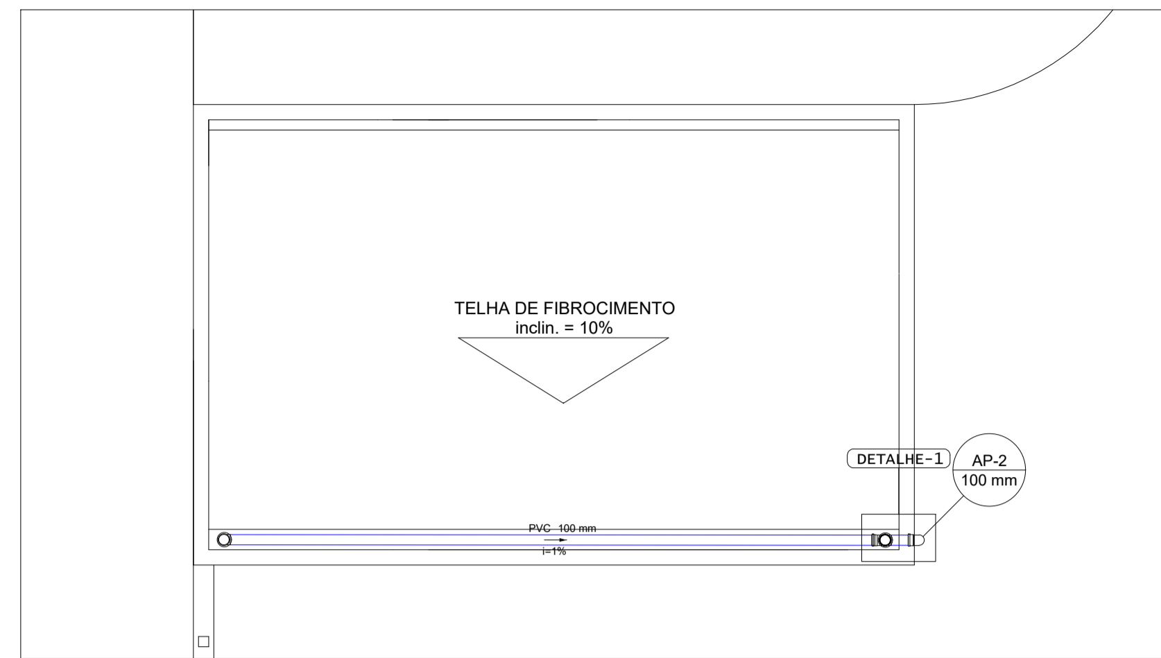
PLANTA DE COBERTURA - RAI-O-X ESCALA 1/50
