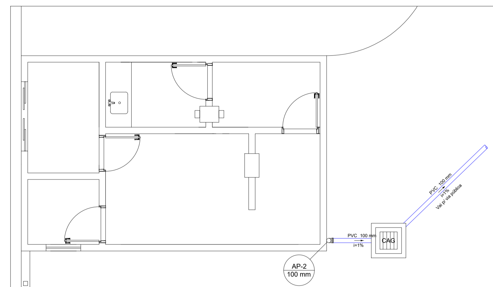
PLANTA BAIXA - RAI-O-X ESCALA 1/50
