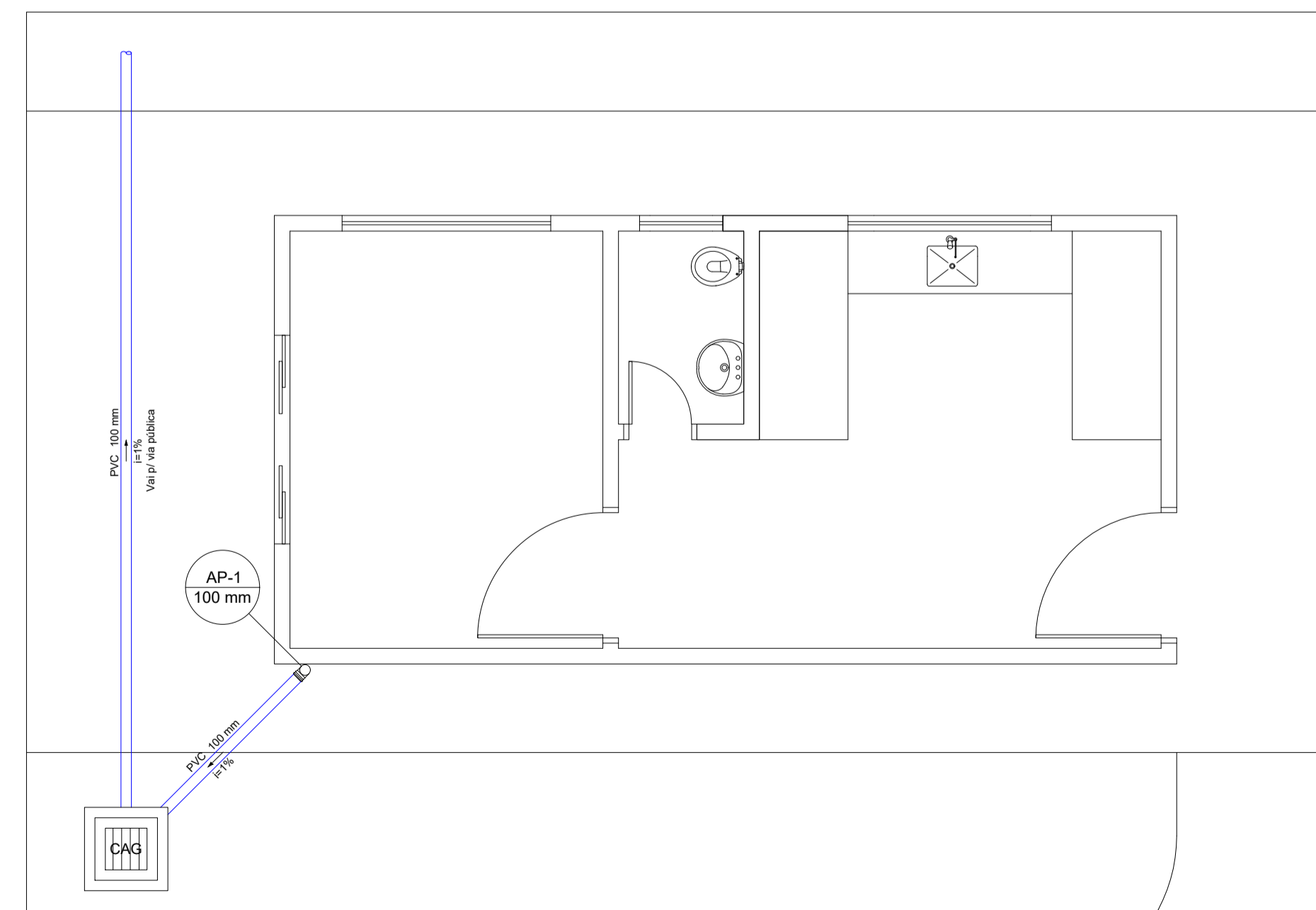
PLANTA BAIXA - NECROTÉRIO ESCALA 1/50
