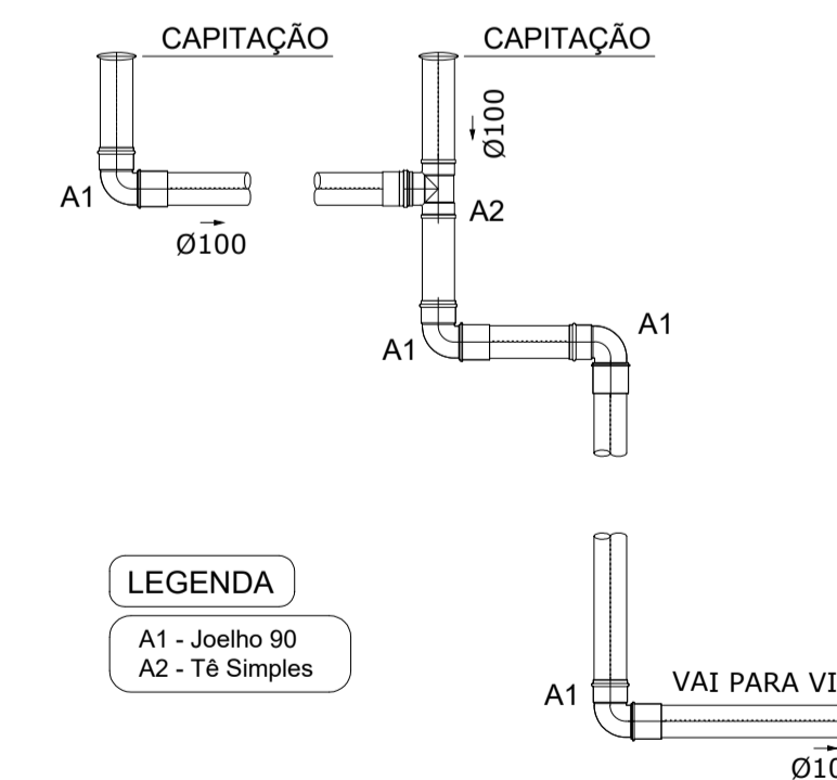
DETALHE 1 ESC. 1:25
