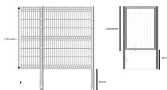
Desenho esquemático dos postes e painéis metálicos e esquemático do portal(portão, coluna e batente)
