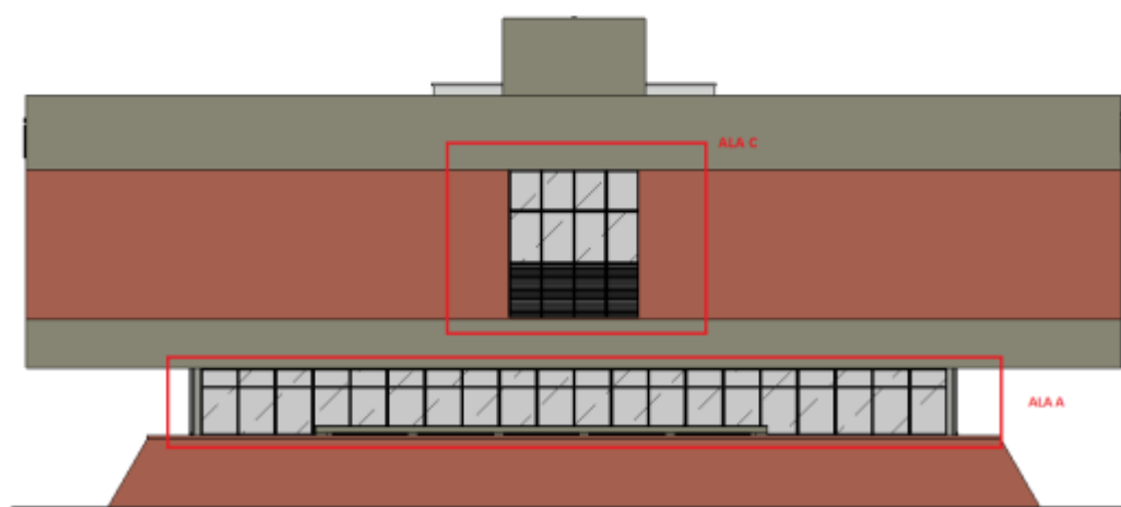
FACHADA OESTE ESCALA: 1 : 125
