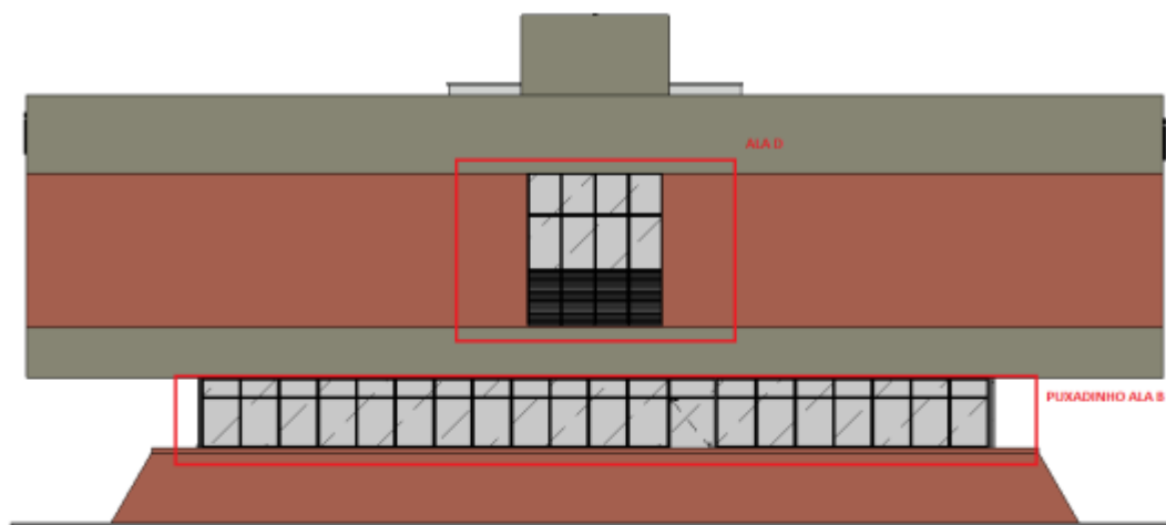
FACHADA LESTE ESCALA: 1 : 125
